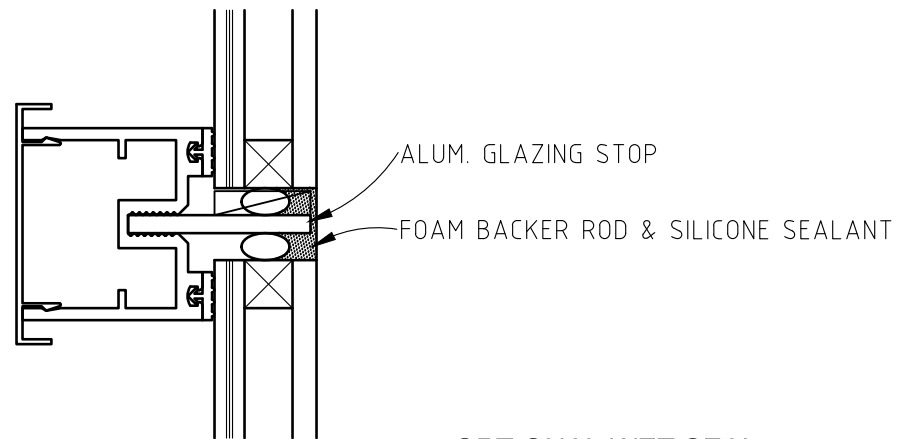
OPTIONAL WET SEAL
